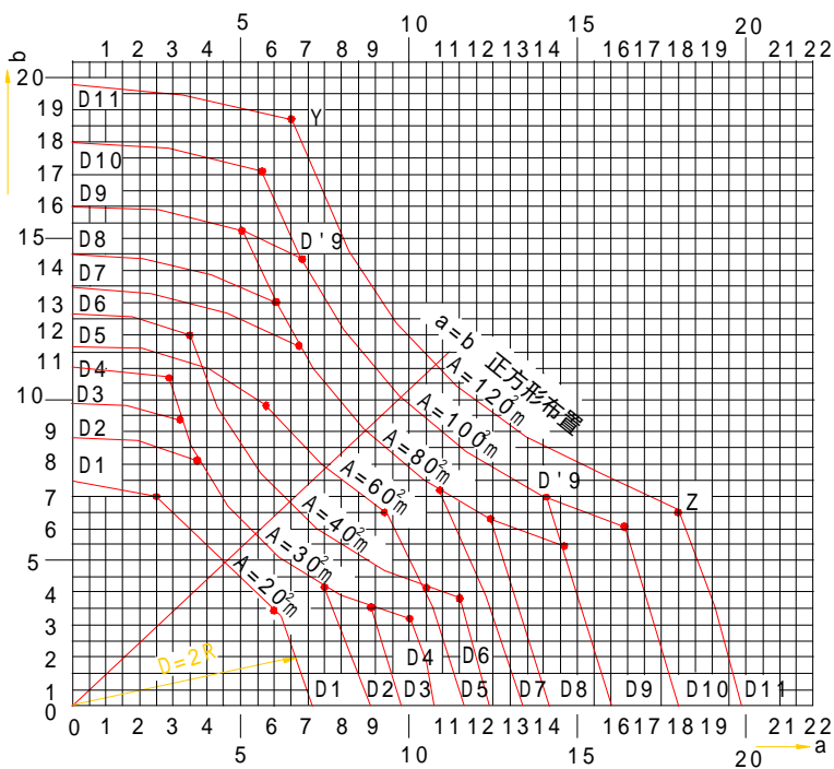
图 A 探测器安装间距的极限曲线
