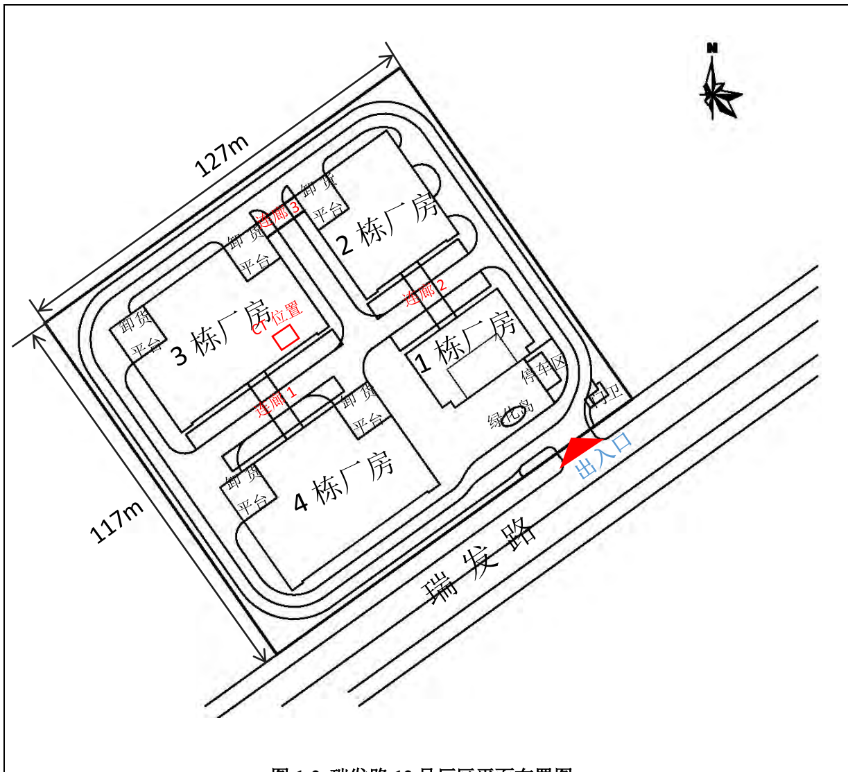
图 1-2 瑞发路 12 号厂区平面布置图
