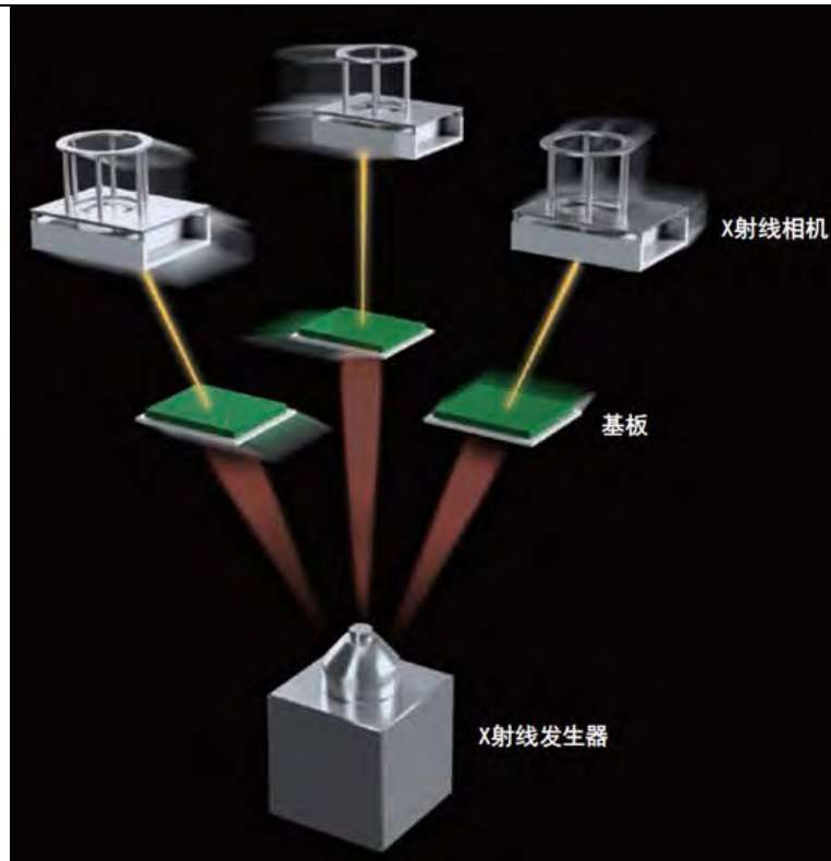
图 9-2 工业 CT 内部构造示意图
