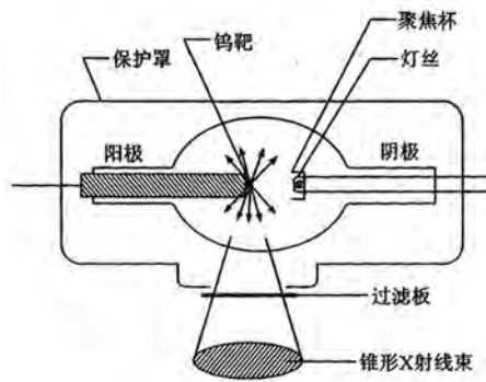
图 9-4 X 射线管示意图
