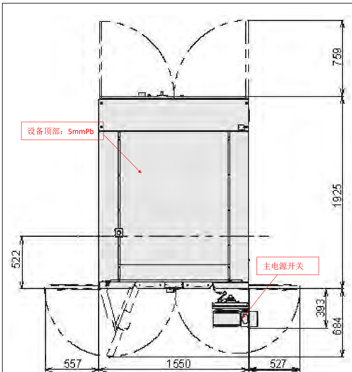
图 10-3 装置结构俯视图
