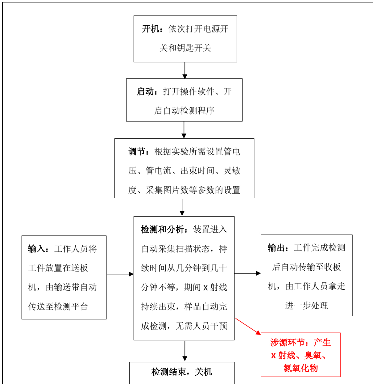
图 9-6 工艺流程及产污环节图
