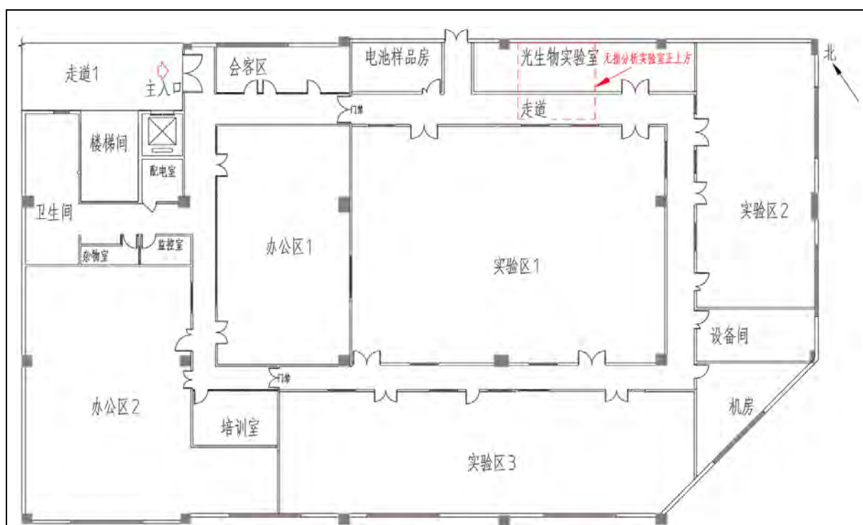
图 2-3 鸿荣源鸿威工业区 C 栋二层平面布置图
