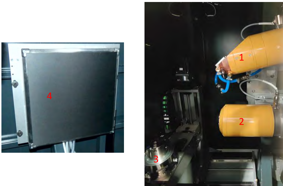
图 2-6 工业 CT 内部结构图
