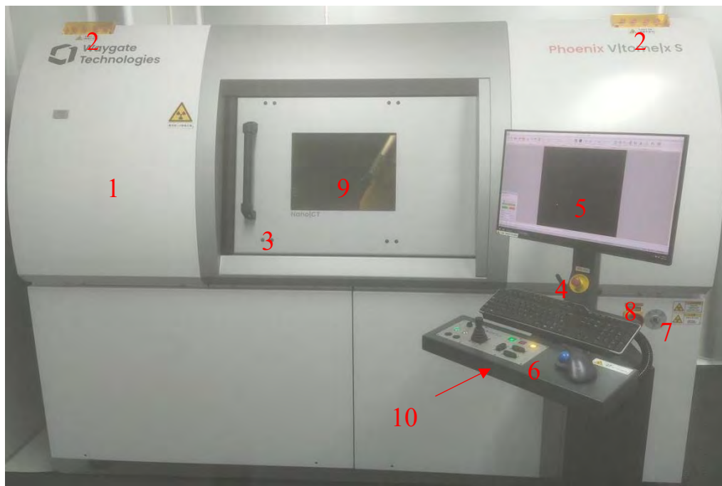
图 2-5 工业 CT 外观结构图
